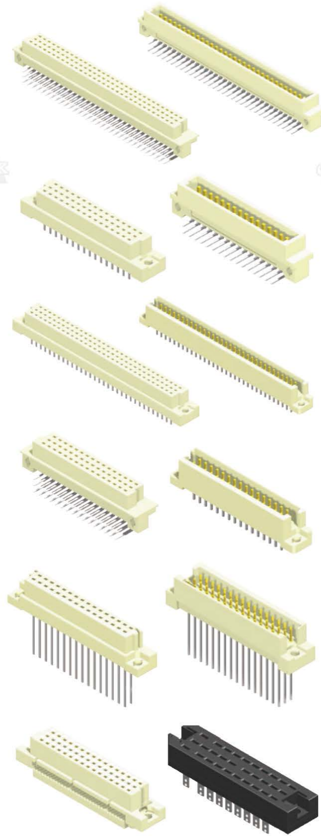
DIN 41612 / 41622
